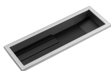
1CVP
